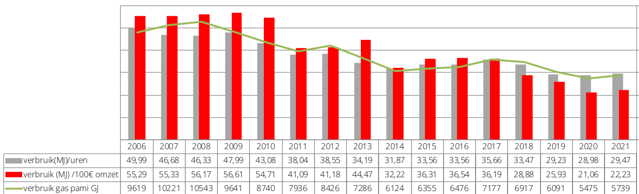
figuur 7.5. gasverbruik Pami (megajoule/jaar)
