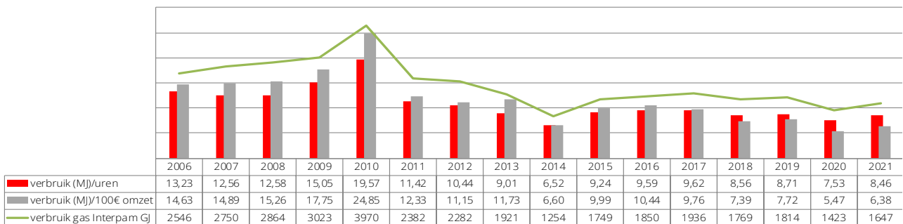
figuur 7.5. gasverbruik Interpam (megajoule/jaar)
