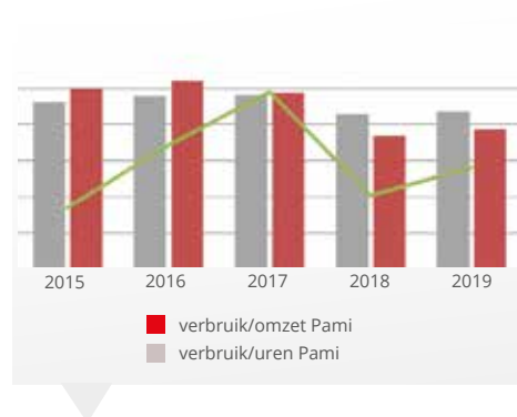
figuur 7.5. gasverbruik Pami (megajoule/jaar)
