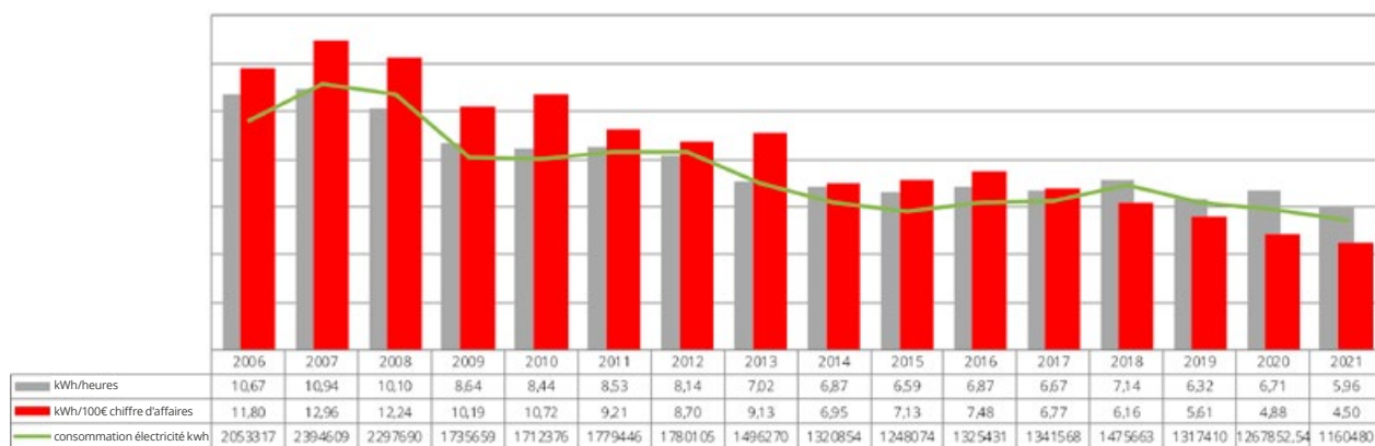
Figure 7.6 - Consommation d'électricité Pami/Interpam (kWh/an)
